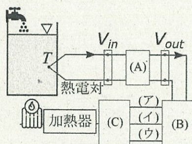
図1 水温制御システム
