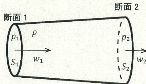
図２ 管路
